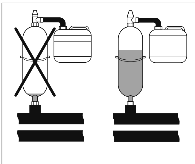
Sl. 6.4 Nivo napolnjenosti izravnalne posode za slano raztopino
