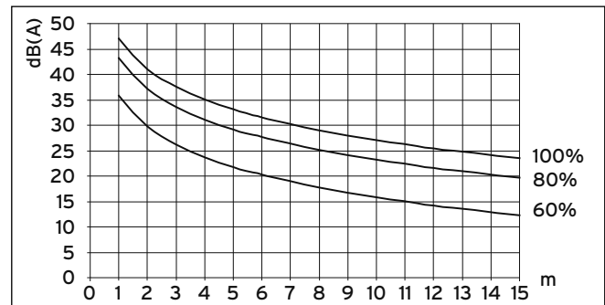
Sl. 6.1 Nivo zvočnega tlaka zunanje enote v dB(A) v odvisnosti od oddaljenosti in števila vrtljajev ventilatorja za VWL 62/3 S pri namestitvi na prostem
