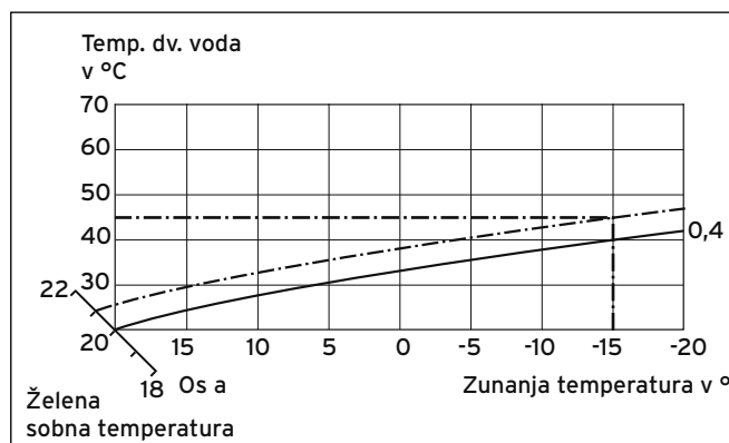
Sl. 2 Vzporedni premik krivulje ogrevanja
