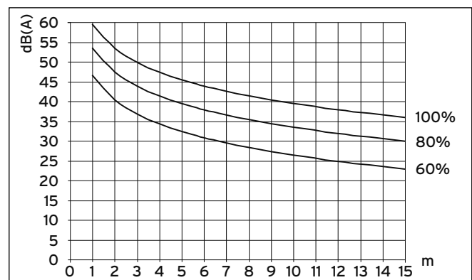
Sl. 6.3 Nivo zvočnega tlaka zunanje enote v dB(A) v odvisnosti od oddaljenosti in števila vrtljajev ventilatorja za VWL 102/3 S pri namestitvi na prostem
