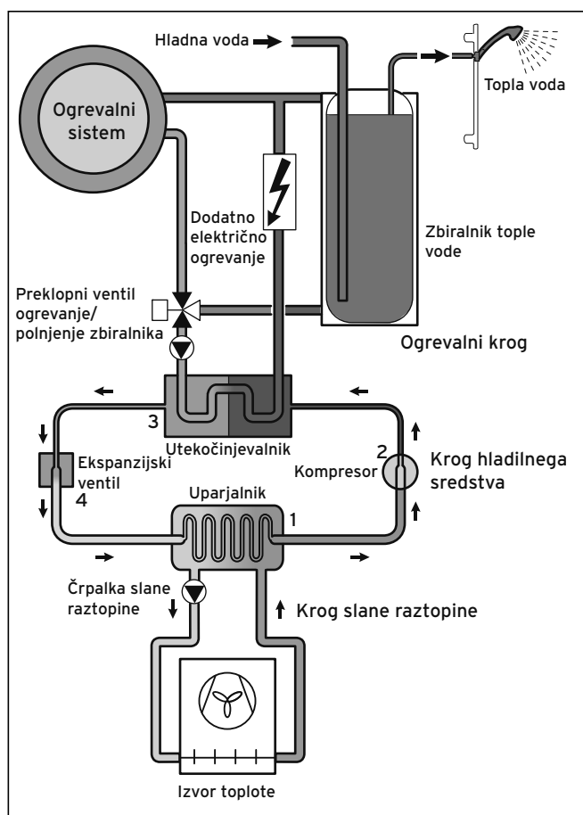
Sl. 3.4 Način delovanja toplotne črpalke
