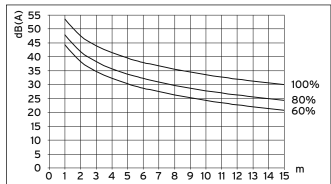
Sl. 6.2 Nivo zvočnega tlaka zunanje enote v dB(A) v odvisnosti od oddaljenosti in števila vrtljajev ventilatorja za VWL 82/3 S pri namestitvi na prostem
